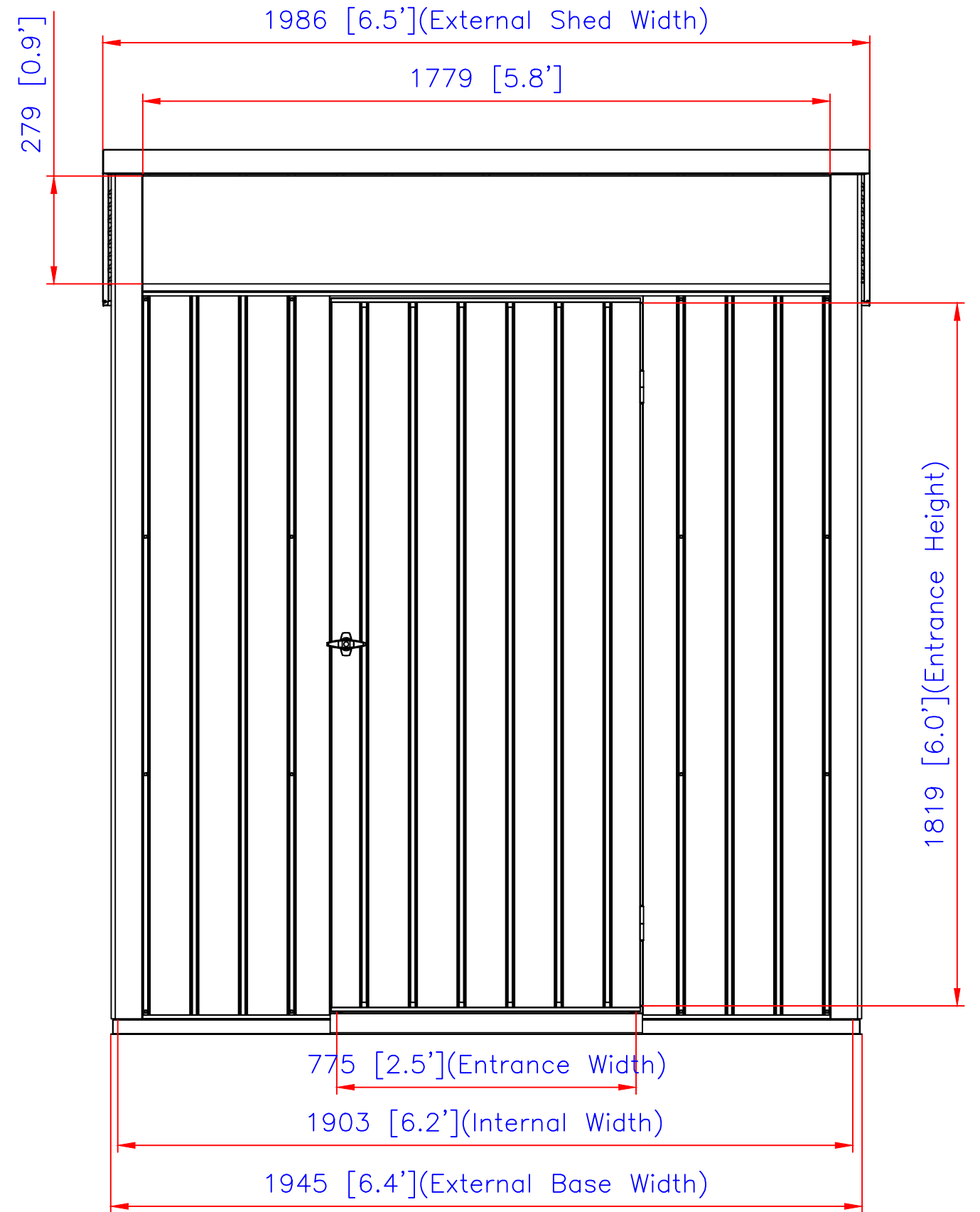
Elevation
