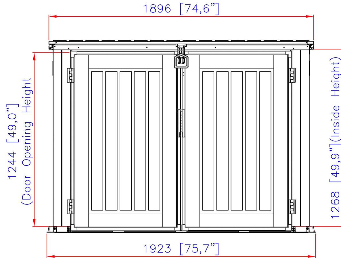
Elevation
