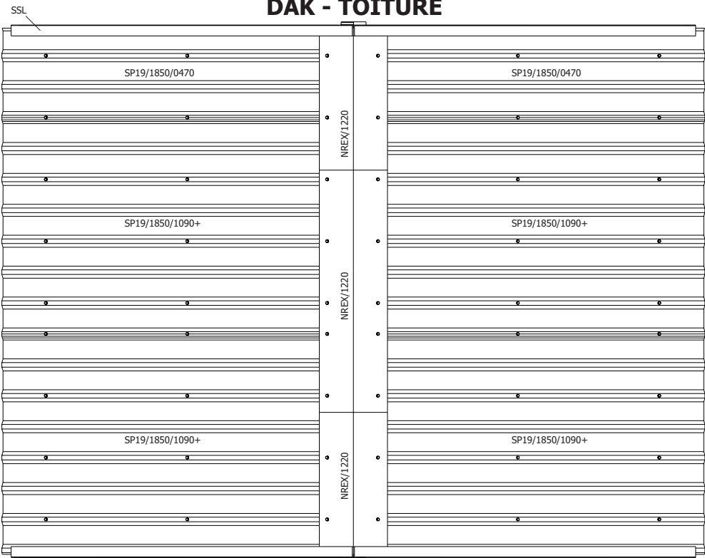
DAK - TOITURE
